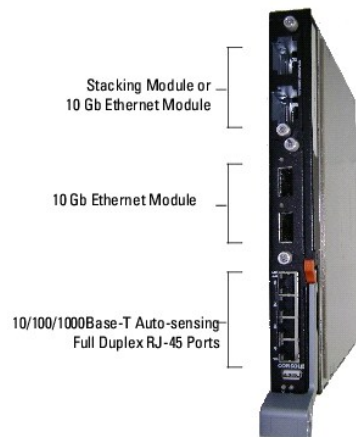
Ilustración 2-1. PowerConnect serie M6220
