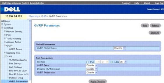
Ilustración 7-62. Parámetros globales de GVRP
