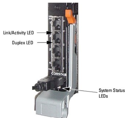
Ilustración 2-3. LED del panel frontal
